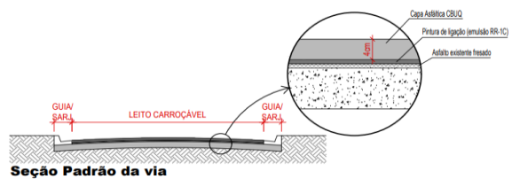
Seção Padrão da via
