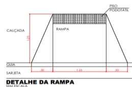
DETALHE DA RAMP
