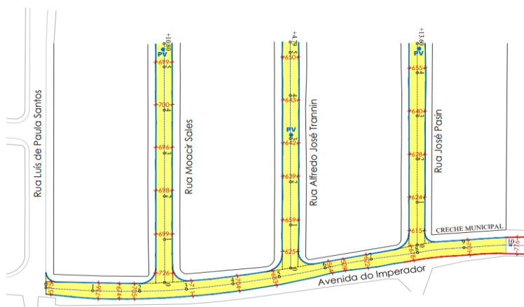
PLANTA DA OBRA TRECHO 1 - ESCALA 1:750
