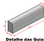
Detalhe das Guias
