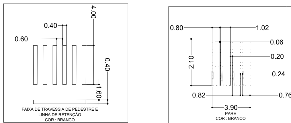
DETALHAMENTO SINALIZAÇÃO HORIZONTAL
