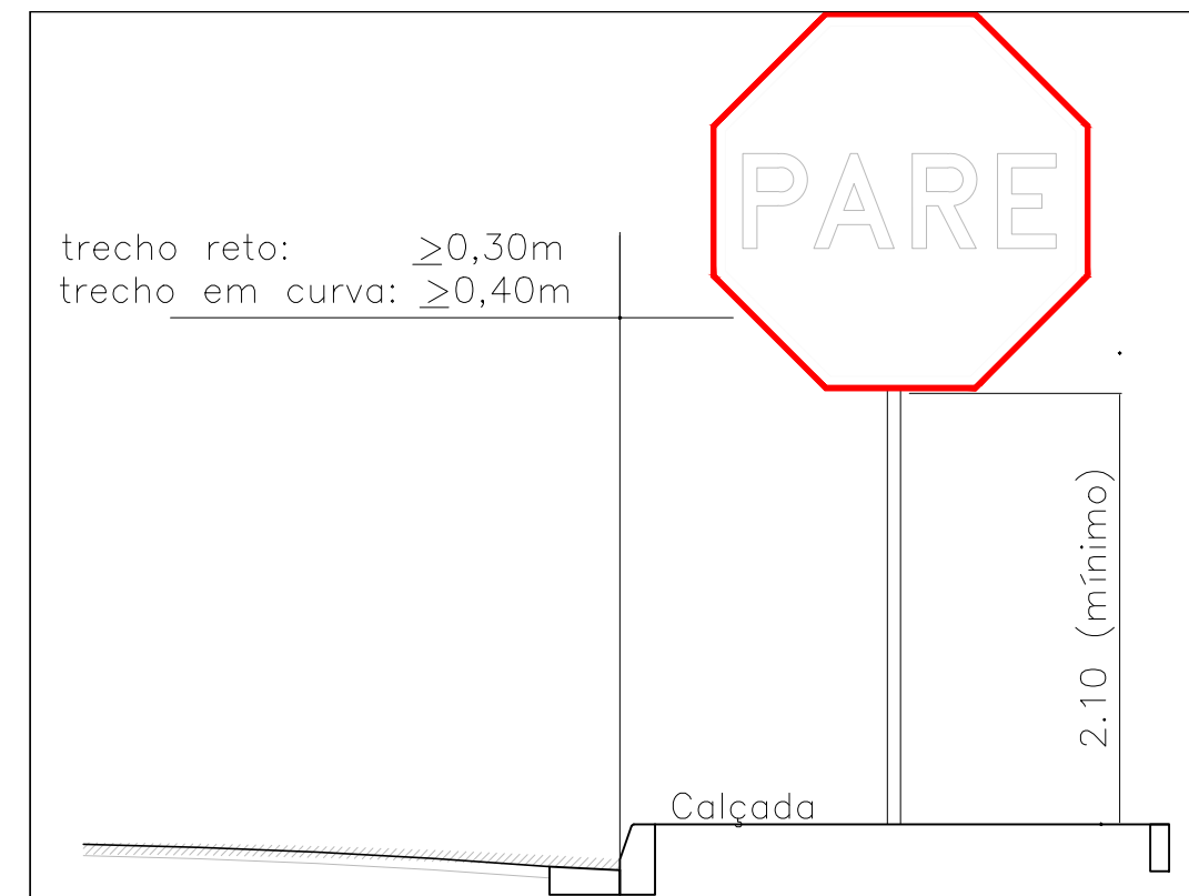
DETALHE IMPLANTAÇÃO DA PLACA
