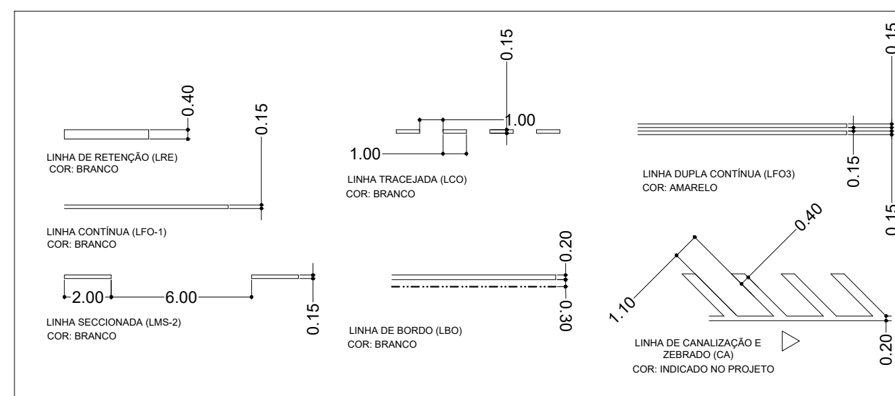
DETALHAMENTO SINALIZAÇÃO HORIZONTAL
