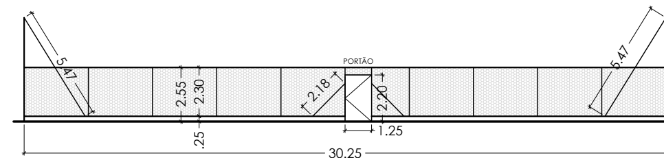
ALAMBRADOS - Vista 04 ESCALA 1 : 250
