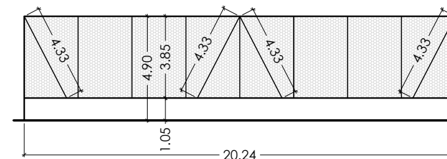
ALAMBRADOS - Vista 01 ESCALA 1 : 250
