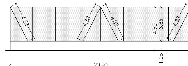
ALAMBRADOS - Vista 03 ESCALA 1 : 250
